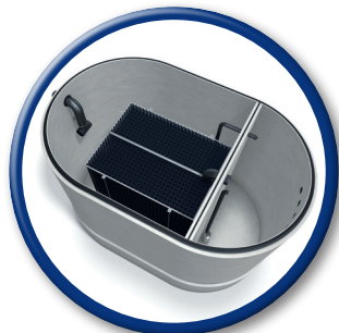
BELEBUNGSBECKEN
